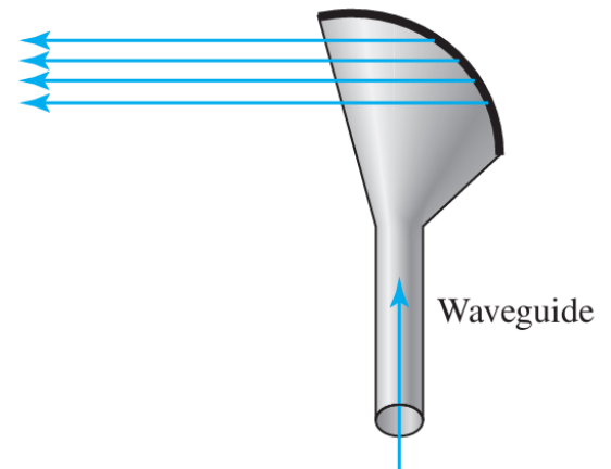
b. Horn antenna
